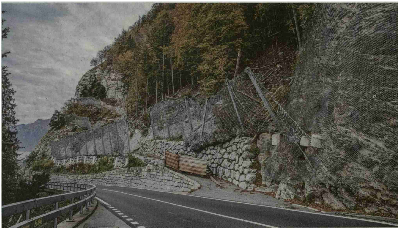
Das Schutznetz hat die Steine des Felsschlags zurückgehalten.
