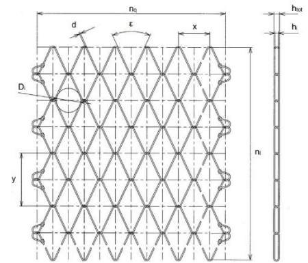
d = 3mm, D i = 65 mm Zugfestigkeit strength 140 kN/m
