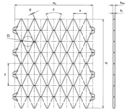
d = 3mm, Di = 80 mm Tensile strength 120 kN/m
